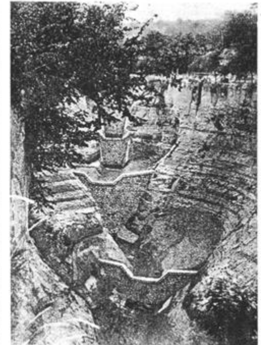
14. kép. A XII., XI. és X. sz. gátak felül- A IX., X. és XI. gát a jobb partról nézve
